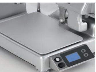
Applicazione bilancia: Pesata max Kg 10 - precisione gr. 2 piatto smontabile, formato mm 225x360
